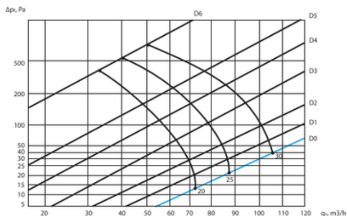
RONDO 100 (odtah vzduchu)
