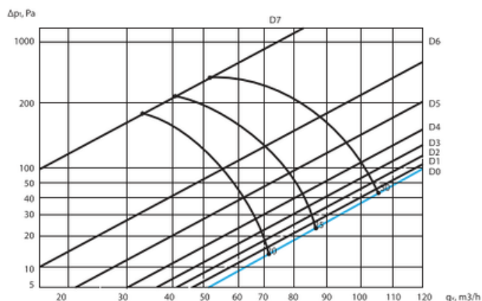
RONDO 125 (odtah vzduchu)
