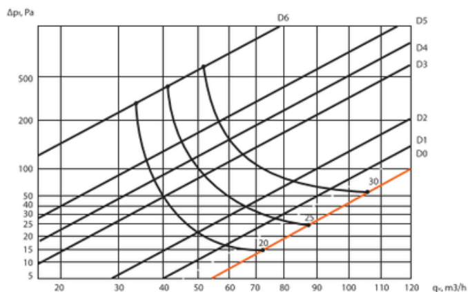
RONDO 100 (přívod vzduchu)
