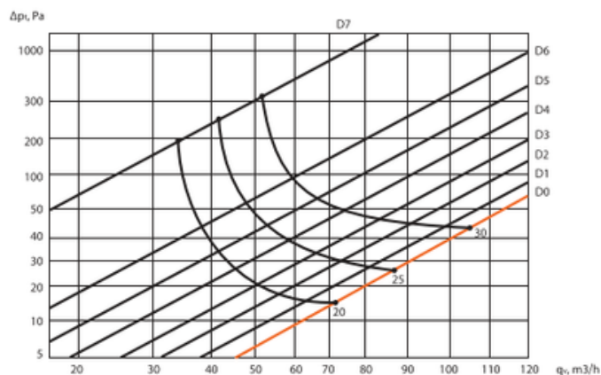
RONDO 125 (přívod vzduchu)
